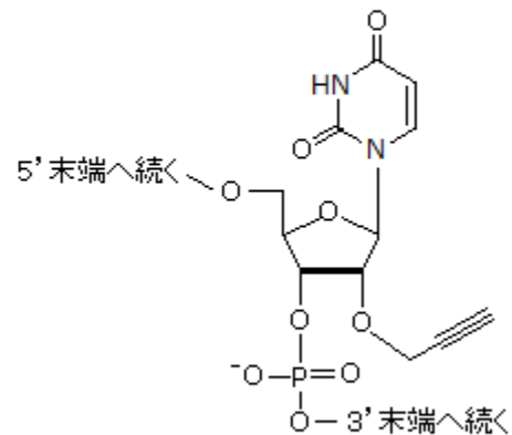
2'-O-propargyl rU
