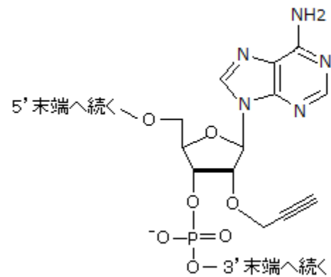
2'-O-propargyl rA
