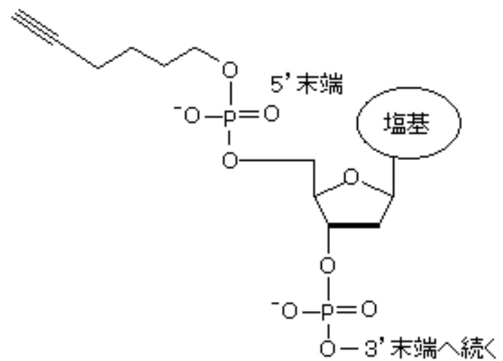
【5'アルキン (Alkyne) 構造式】
