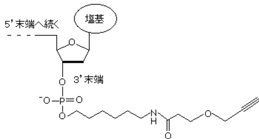
【3'アルキン (Alkyne) 構造式】
