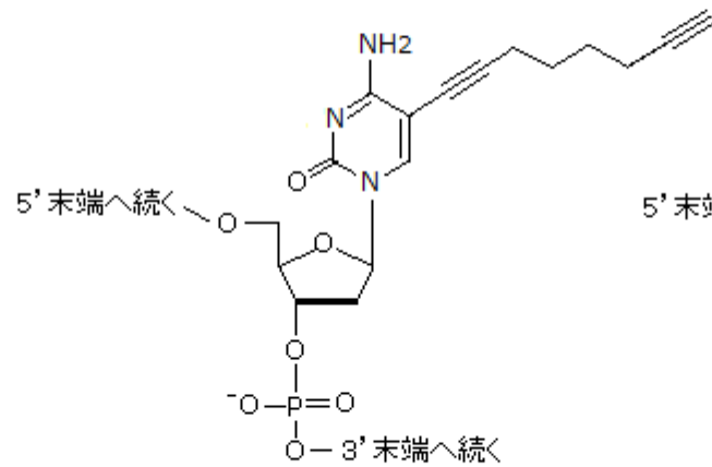
C8-alkyne-dC (5-Octadiynyl-dC)
